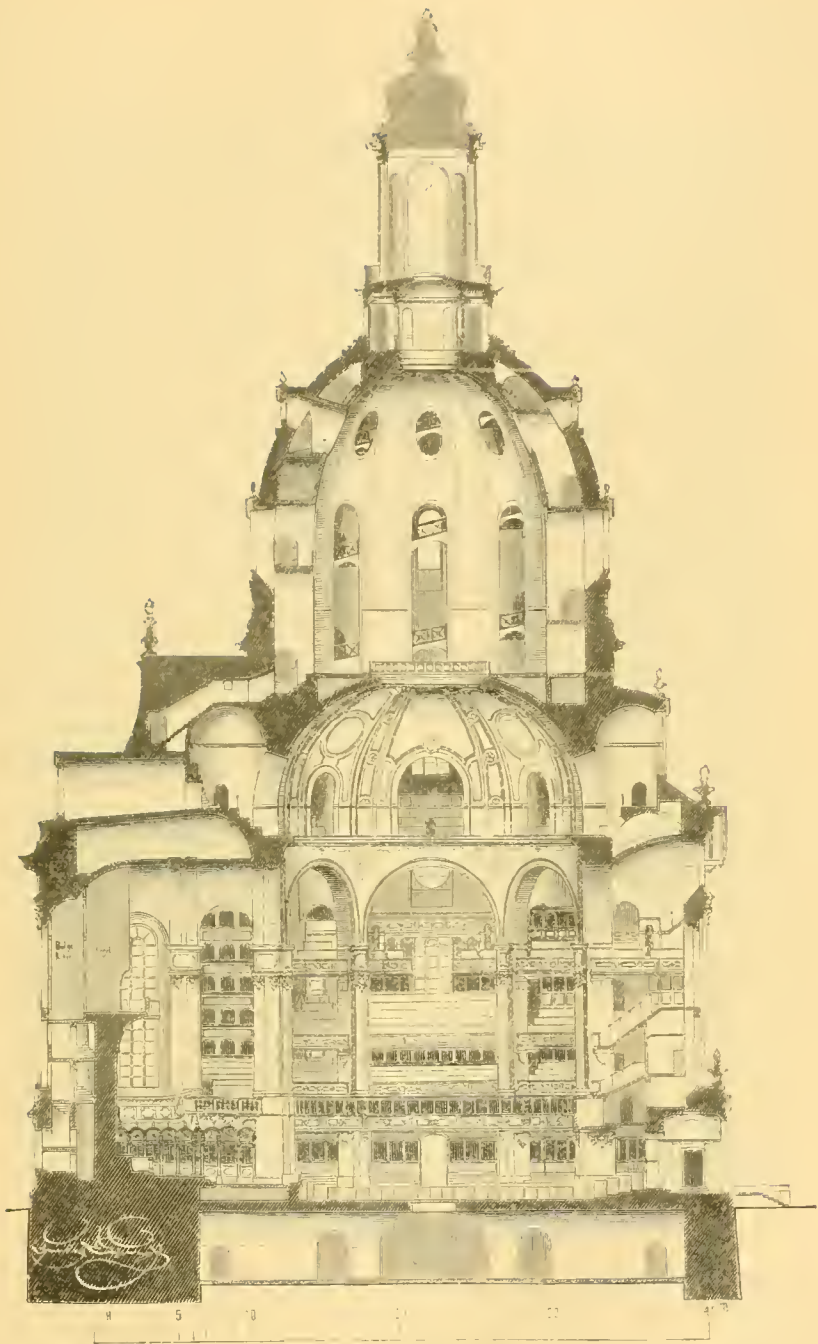
Fig. 21. Frauenkirche zu Dresden. Längsschnitt.
